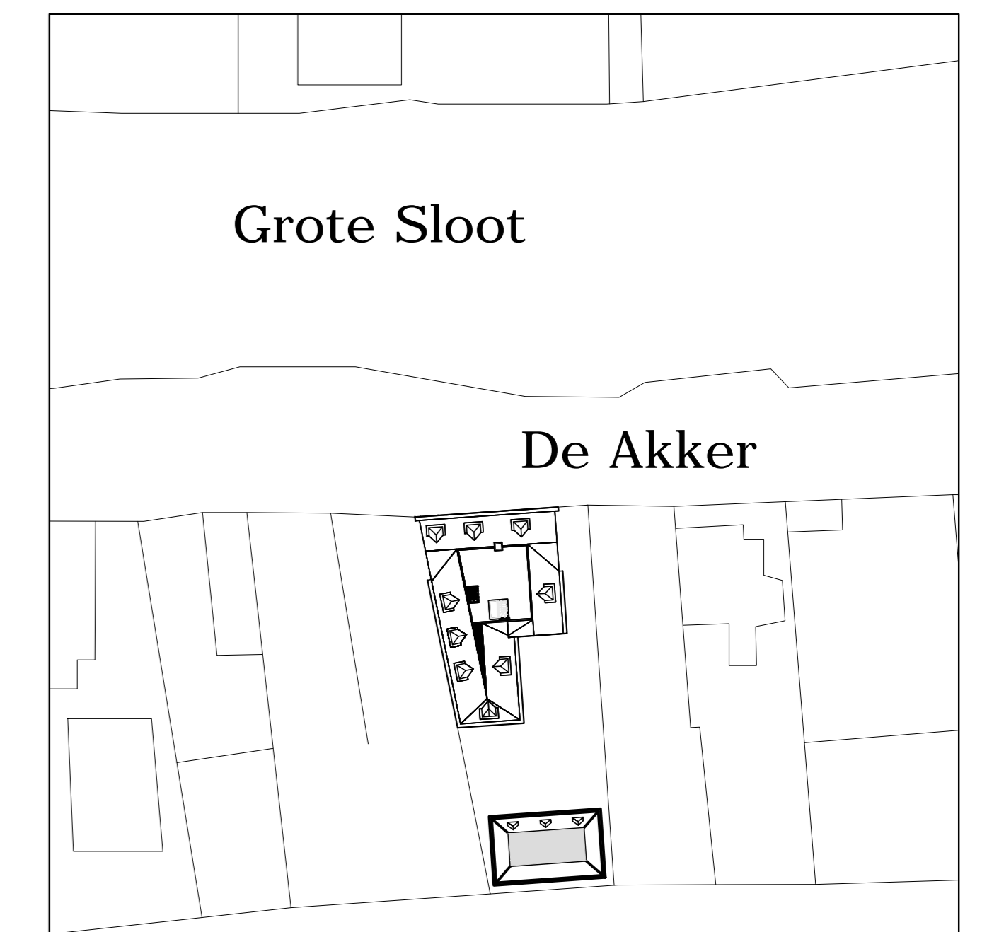
nieuwe situatie
