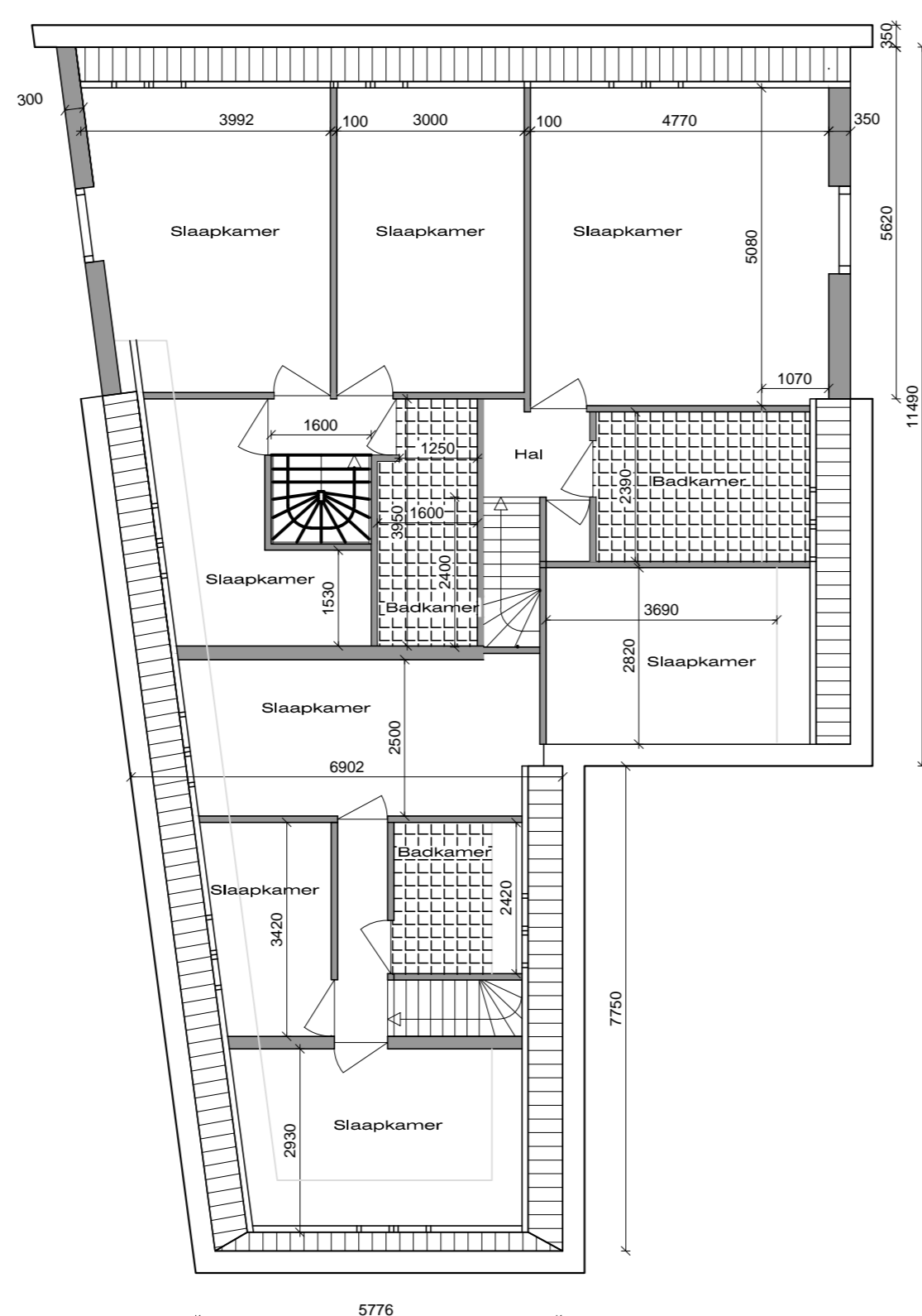
Eerste verdieping
