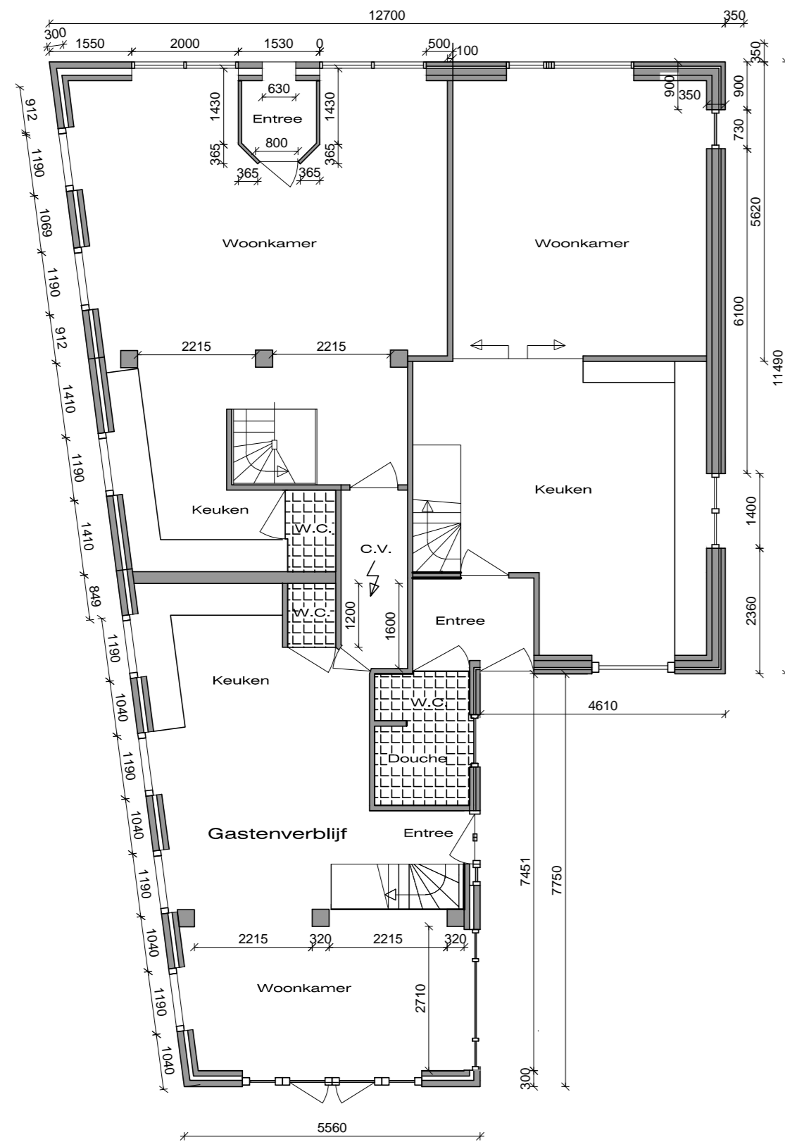
Begane grond
