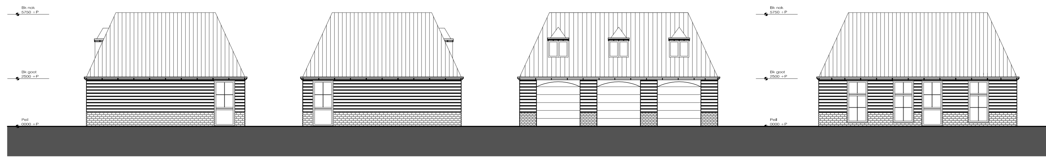
Noordgevel nieuw
